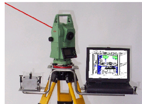
Lasermess-Station „CASOB®-Rohr“
